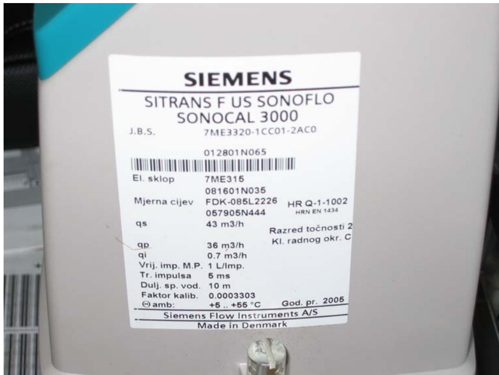
Slika 3a: Natpisne pločice mjerila protoka mjerila toplinske energije SITRANS F US SONOFLO SONOCAL 3000/3300
